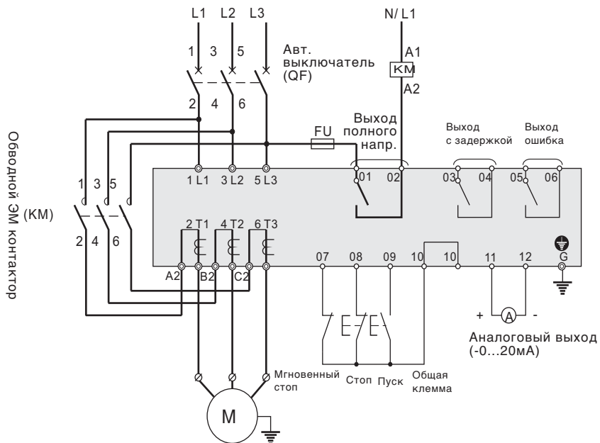
2-9 Схема подключения реле и пульта управления
